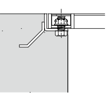
■ ボルト固定断面図
