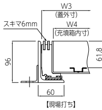
■ 断面図
