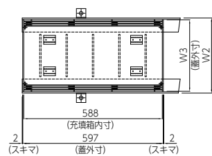
■ 平面図
