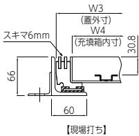
■ 断面図
